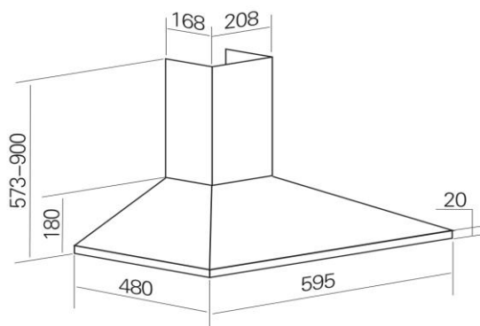
Einbauskizze
